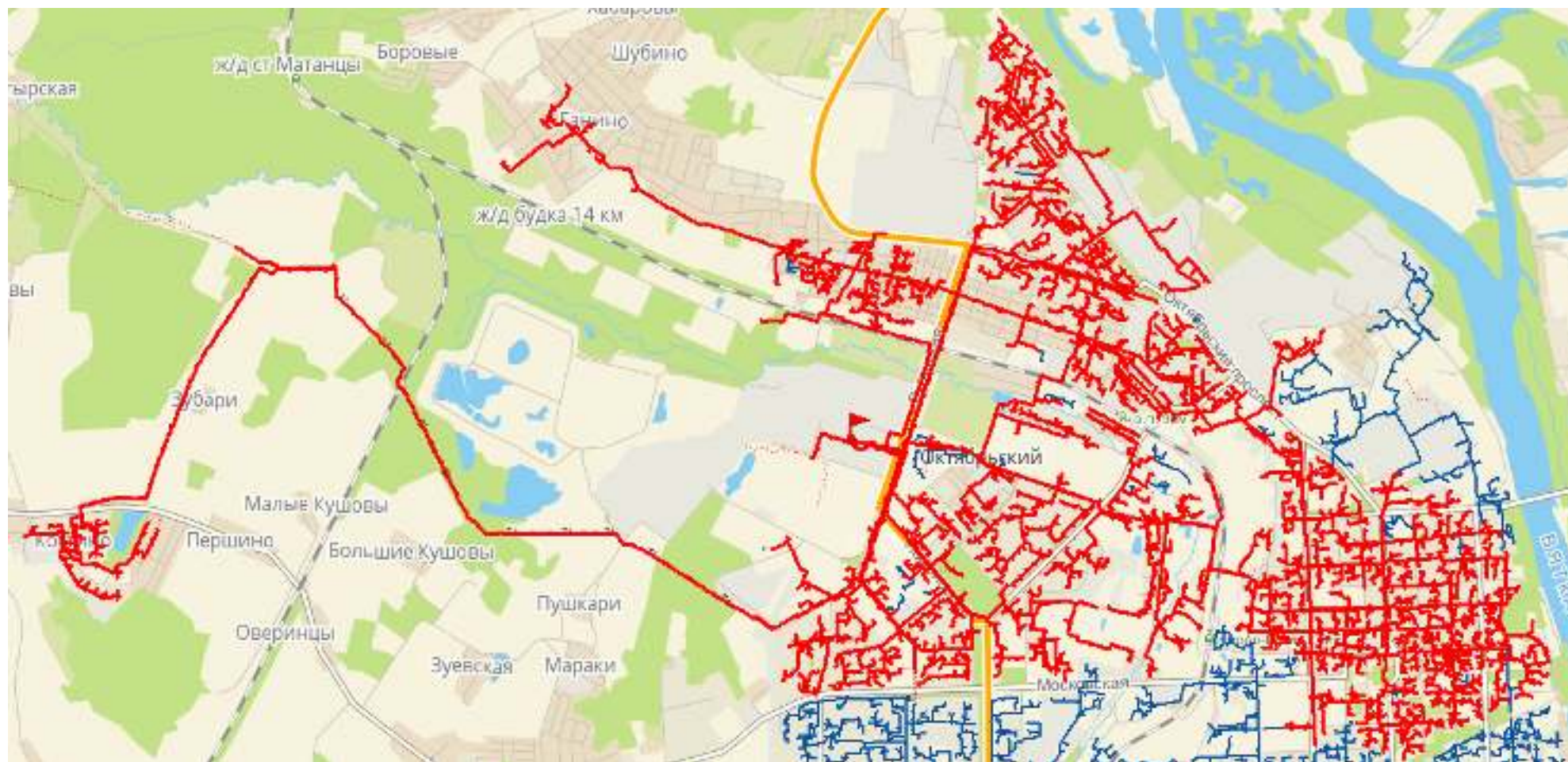
Рис. 2.1 Тепловая сеть ТЭЦ-4
