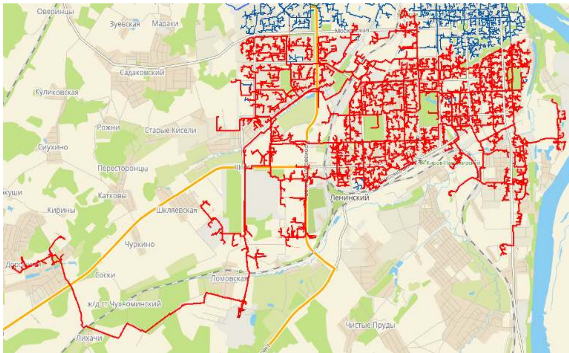
Рис. 3.1 Тепловая сеть ТЭЦ-5
