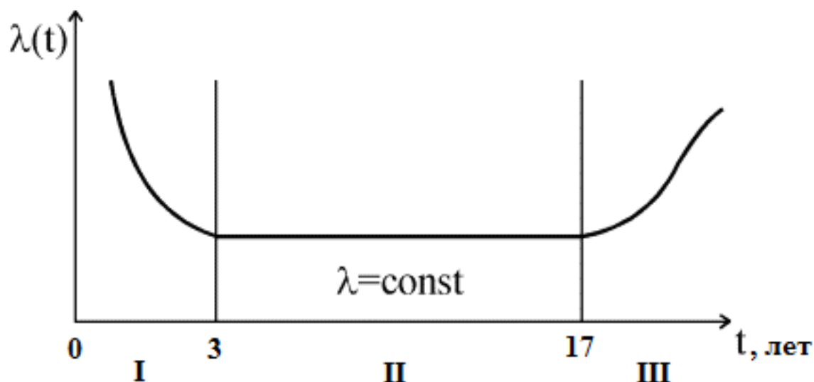
Рис. 1.2 Интенсивность отказов по кривой распределения Вейбулла I - период приработки и отказов некачественных элементов; II - период нормальной эксплуатации; III - период старения (отказы вызваны старением материалов).
