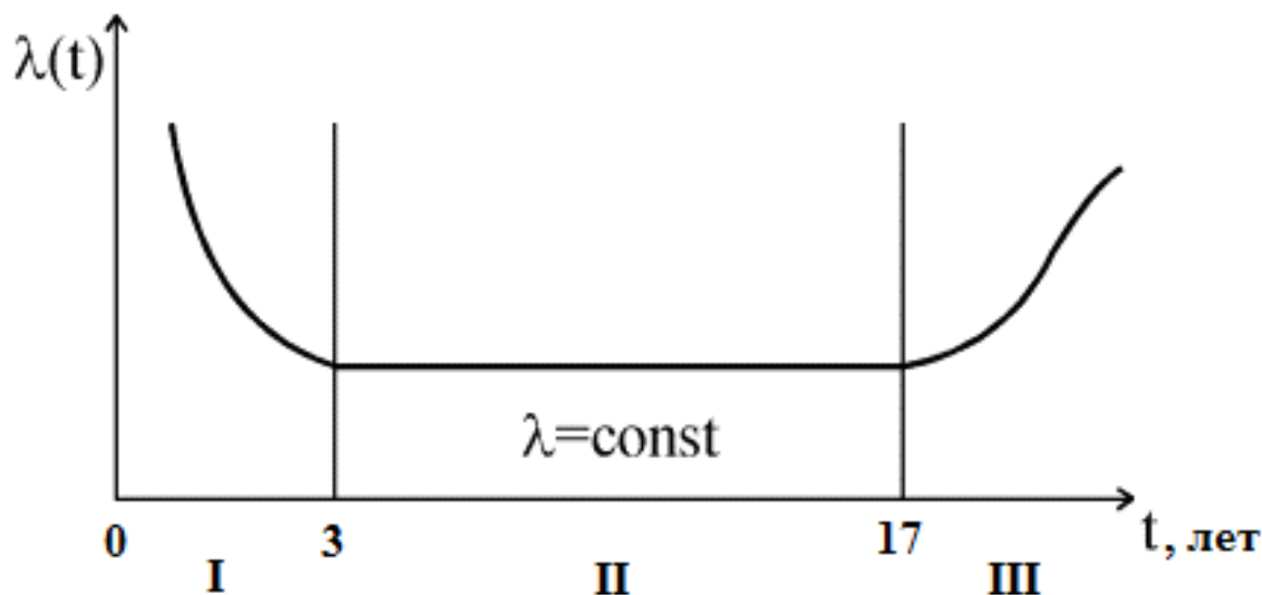
Рис. 3.2 Интенсивность отказов по кривой распределения Вейбулла I - период приработки и отказов некачественных элементов; II - период нормальной эксплуатации; III - период старения (отказы вызваны старением материалов).
