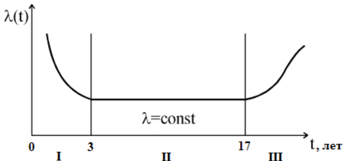
Рис. 1. Интенсивность отказов по кривой распределения Вейбулла I - период приработки и отказов некачественных элементов; II - период нормальной эксплуатации; III - период старения (отказы вызваны старением материалов).
